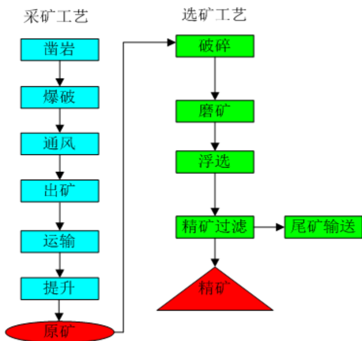
凡口铅锌矿采选工艺流程图
